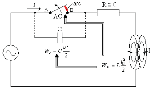
Fig. 0.2 Relativ la întreruperea cu arc electric a unui circuit inductiv
